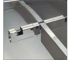
Conjunto de soportes en acero inox para realizar las diferentes composiciones de cubetas en exposición.
